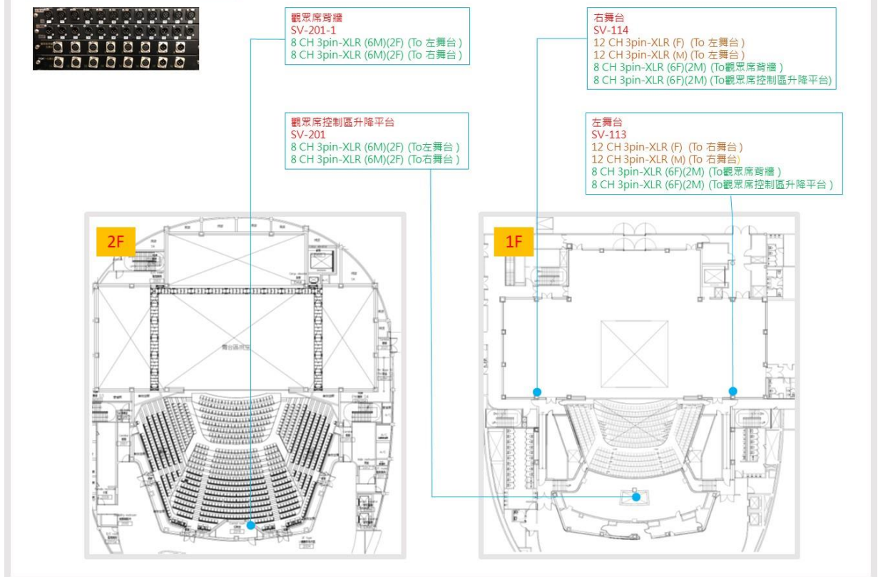
圖例 4-1.7 信號通道圖示
