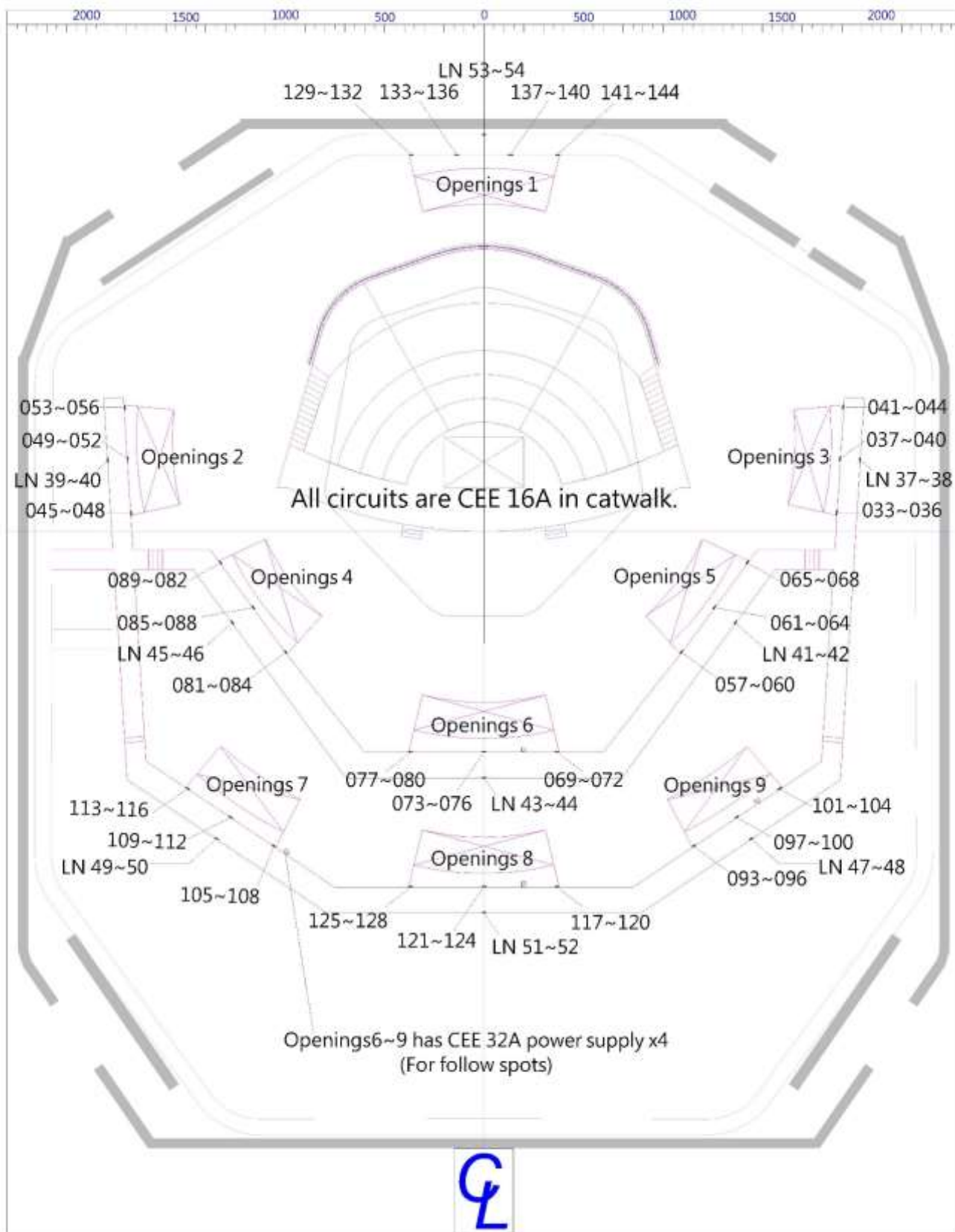
圖例 3.5.2.1- 外區燈光迴路配置
