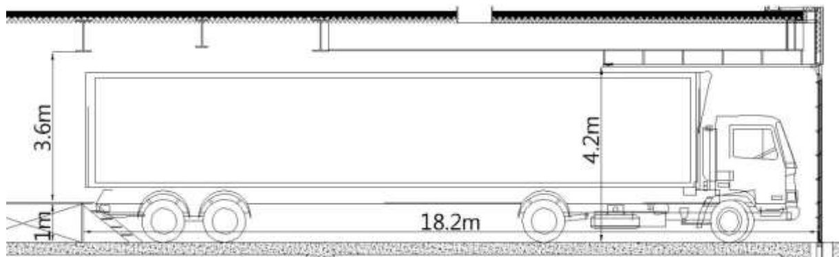
圖例 5.2 東碼頭卸貨口剖面圖
