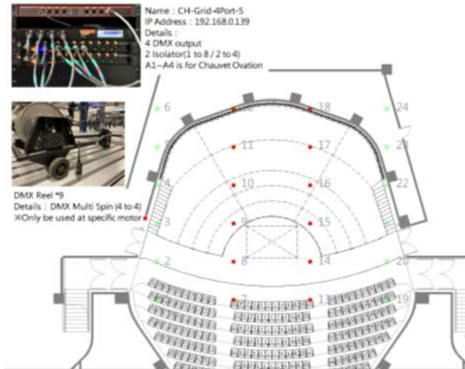
圖例 3.4.1- 頂棚區 Node 位置圖
