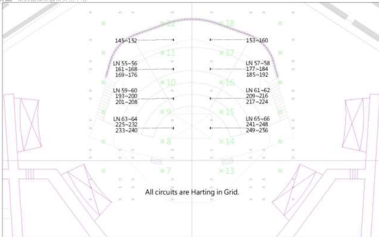
圖例 3.5.2- 舞台頂棚區燈光迴路配置
